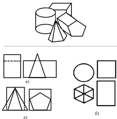
Сурет 12- Үш проекцияда көрсетілген объекттер
