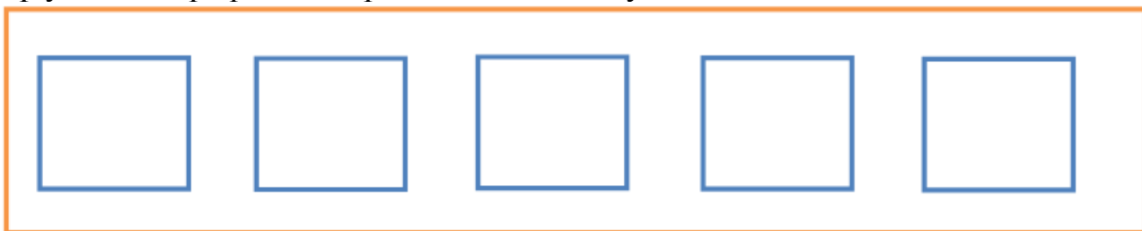
Сурет 10.1 – Шаршылар
