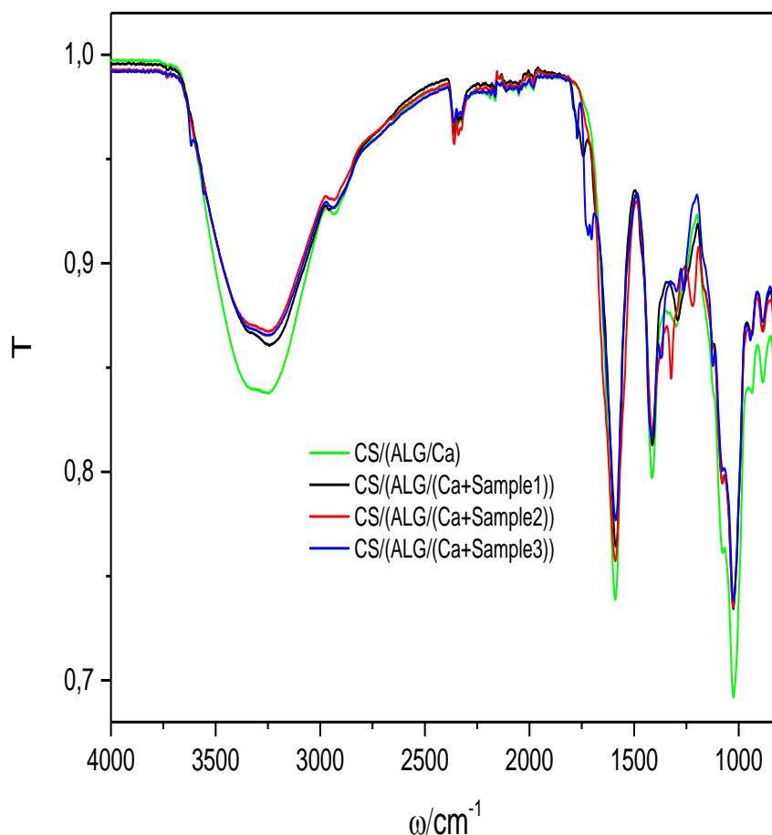
Сурет 12 - FTIR сипаттамасы-құрғақ микрокапсулалар құрамдарының спектрі: CS/(ALG/Ca) (жасыл сызық), (CS/(ALG/(Ca+ Үлгі№1))) (қара сызық), (CS/(ALG/(Ca+Үлгі№2))) (қызыл сызық), (CS/(ALG/(Ca+Үлгі№3))) (көк сызық);
