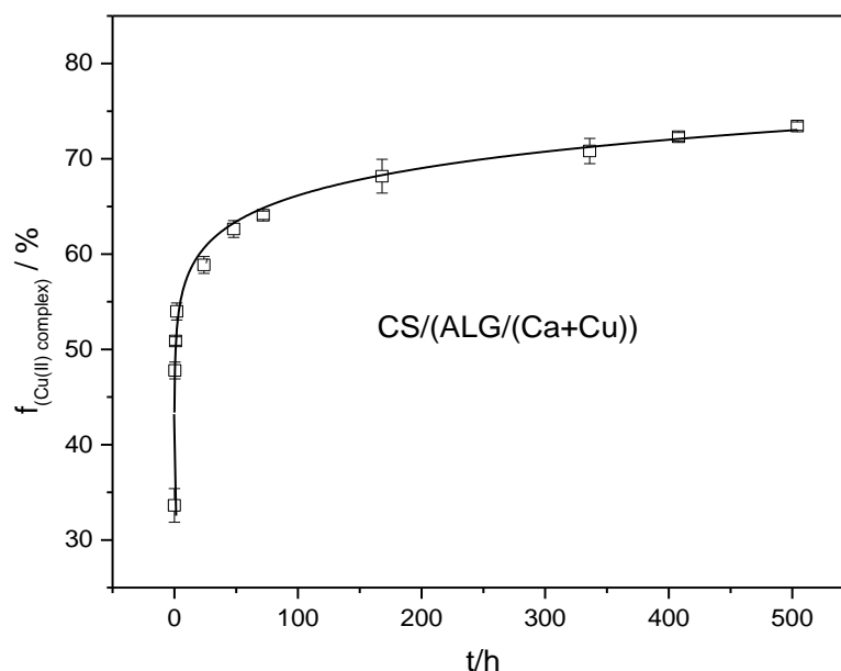
Сурет 20 - Кальций хлоридінің бастапқы концентрациясында дайындалған CS/(ALG/(Ca+Cu/үлгі№5)) микрокапсулаларынан уақыт өте бөлінген мыс (II) кешенінің пайызы, W(\text{CaCl}_2)/\% = 1 (құрамында 1,5% ерітілген мыс (II) кешені/үлгі№5 бар).
