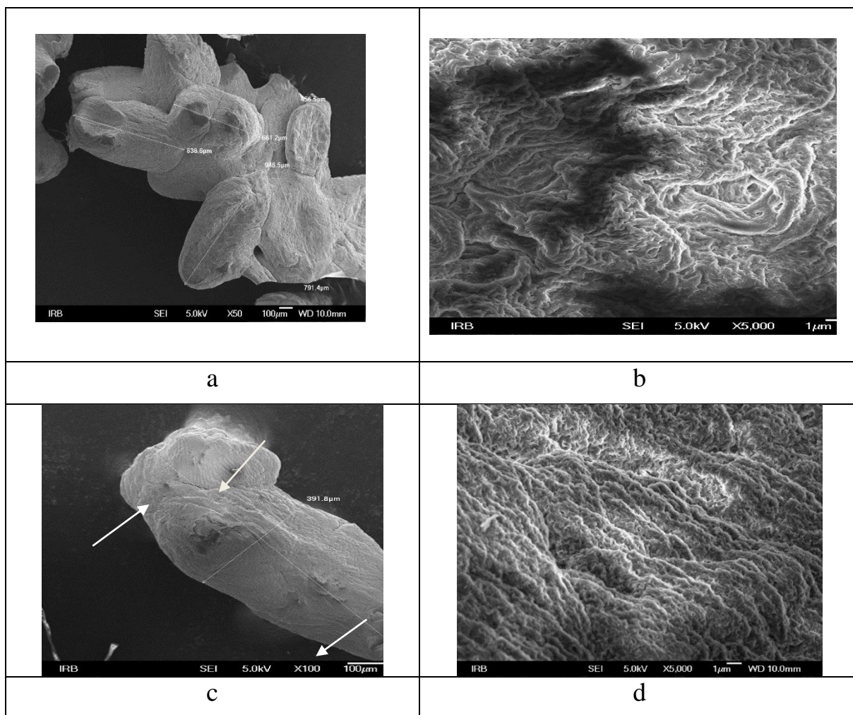
Сурет 17 - Сканерлеуші электронды микроскоптың көмегімен (a, b) CS/(ALG/Ca) б (C,d) CS/(ALG/Ca+Cu/үлгі№5)) кальций хлоридінің бастапқы концентрациясында дайындалған кептірілген микрокапсулалар, w(\text{CaCl}_2) / \% = 1 (құрамында 1,5% ерітілген мыс (II) кешені бар). Бағандар белгіленген.
