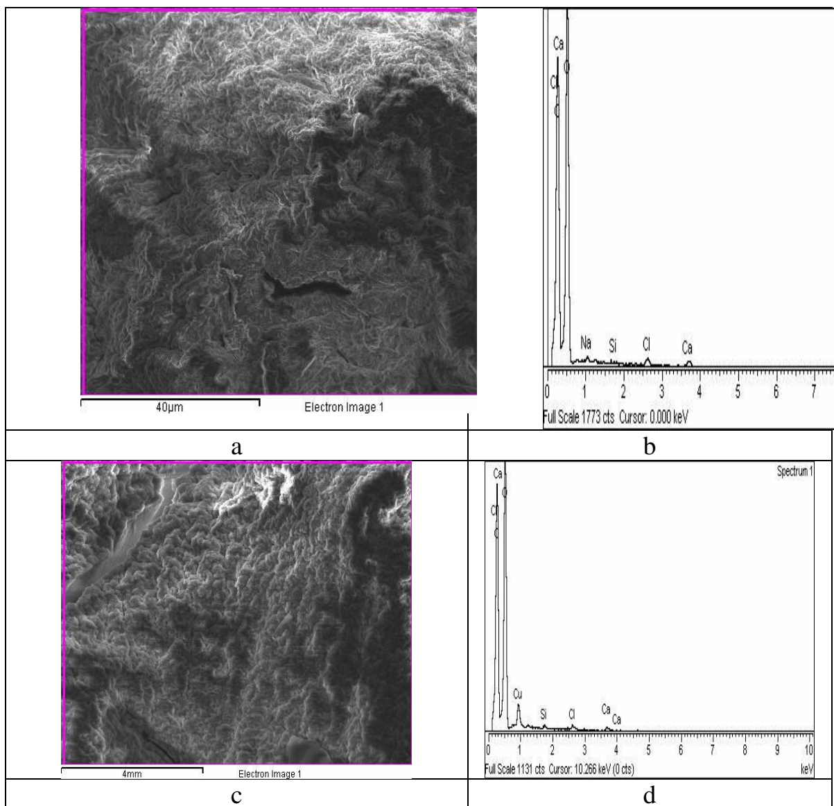
Сурет 18 - Микрокапсулалардың беткі морфологиясы (a) CS/(ALG/Ca) және (c) CS/(ALG/(Ca+Cu/үлгі№5)) және элементтік беттік талдау (%) (b) CS/(ALG/Ca) және (d) дисперсиялық рентген спектроскопиясын (EDX) қолданып CS/(ALG / (Ca+Cu/үлгі№5)). Микрокапсулалар кальций хлоридінің бастапқы концентрациясында дайындалды, w(\text{CaCl}_2) / \% = 1 (құрамында 1,5% ерітілген мыс (II) кешені бар). Бағандар белгіленген
