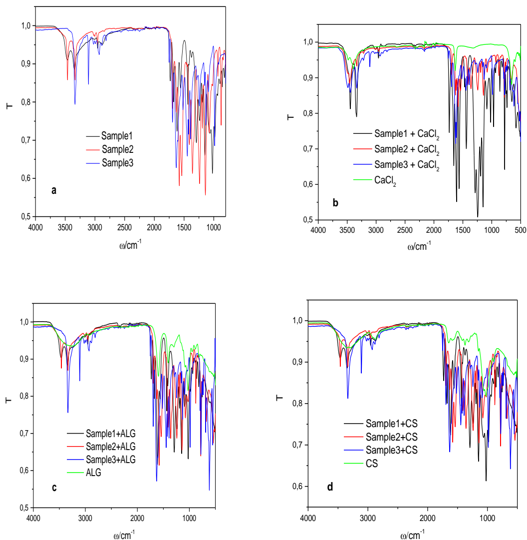
Сурет 11 - FTIR-спектр: (a) үлгі 1(қара сызық), үлгі 2 (қызыл сызық) және үлгі 3 (көк сызық), (b)кальций хлориді \text{CaCl}_2 қоспасы, (c) ALG (қара сызық) қоспасы, (d) хитозан CS қоспасы. Қосылған \text{CaCl}_2 , натрий альгинат (ALG) және хитозан (CS) спектрлері жасыл сызықтармен көрсетілген
