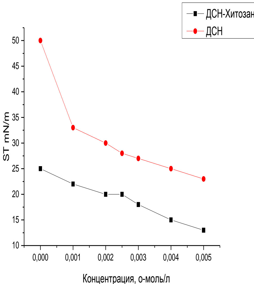
Сурет 4 - Тепе-теңдіктегі беттік керілу ерітінді концентрациясының функциясы ретінде (ДСН ерітіндісі, ДСН-Хитозан кешені). Хитозанмен бірге ДСН ерітіндісінің концентрациясы тұрақты болып таңдалды ( 10^{-2} моль/л)
