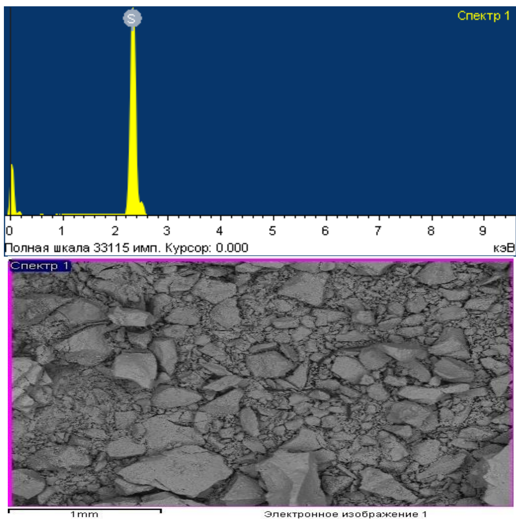
Сурет 9 - Тенгіз күкіртінің электрондық микросуреті және энергодисперсиялық микроталдау нәтижелері
