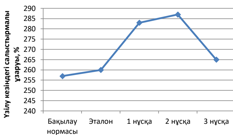
Сурет 13 - Вулканизаттардың созылу кезіндегі салыстырмалы ұзаруы
