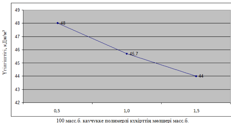
Сурет 10 - Протекторлы резеңкелердің физикалық-химиялық қасиеттерінің күкірт мөлшеріне тәуелділігі
